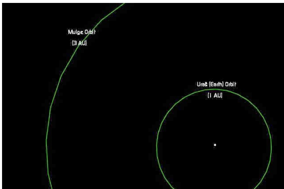
Figura. MMTV1. Vista al plano elíptico mostrando las orbitas de Uraś (Tierra) y Mulge. A esta escala, los planetas mismos no son visibles, ni sería visible el sol, excepto por el hecho de que es auto-luminoso. Nosotros mostramos al Sol como un punto plano, no a escala. Las torceduras en las órbitas son un artefacto gráfico.
