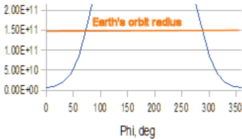
Fig. MMTV-6. Perihelio de la órbita de Mulge-Tab (metros) contra grado \phi . El radio de la órbita de Mercurio es ~50 millones de kilómetros (5.00 E+10). Para los valores de \phi < \pm 20 grados, Mulge-Tab puede llegar más bien algo cerca del sol (véase la tabla arriba), cuyo radio de la fotosfera es de 0.7 millones de kilómetros.
