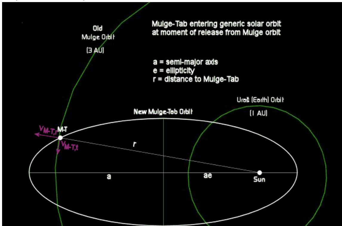
Fig. MMTV-4. Diagrama simplificado de Mulge-Tab en el momento del lanzamiento de la órbita de Mulge, entrando a la órbita genérica elíptica solar.
