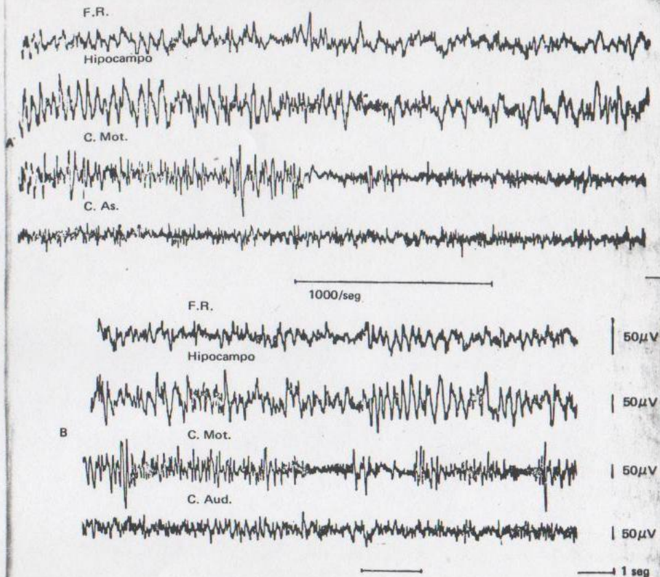
FIG. 3.4 A: la primera aplicación de un sonido indiferente (1000 cps) desincroniza la actividad neocortical e hipocámpica B: Un sonido familiar (puss, shuu) provoca actividad sincrónica en el hipocampo. (Tomado de Lissak y Grastyán, 1960.)
