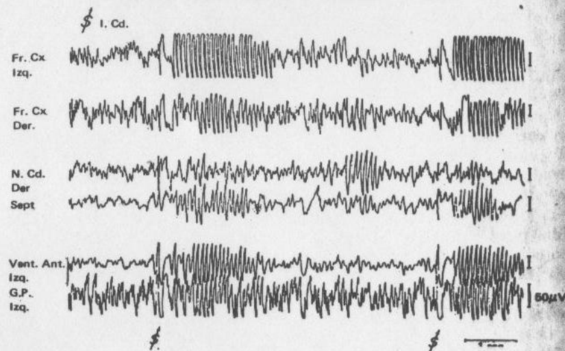
FIG. 2.6 La estimulación del núcleo caudado (70 volts, 0.01 msec. de duración y 5 seg. de intervalo) provoca la aparición de usos en la corteza. $ I. Cd.: estimulación del núcleo caudado izquierdo; Sept.: septum; Vent.: Ant. núcleo ventral anterior del tálamo; G.P.: Globus pallidus; Fr. Cx circunvolución sigmoidea anterior. (Tomado de Buchwald y colaboradores, 1961.)
