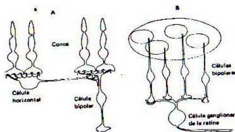
FIG. 4.9 Probable explicación anatómica del mecanismo fisiológico responsable de la direccionalidad selectiva. En A una célula bipolar recibe información convergente excitatoria de un grupo de conos y es inhibida, a través de una célula horizontal, por un segundo grupo de conos desplazados lateralmente con respecto al primero. La secuencia de iluminación de las dos poblaciones de conos determina la selectividad direccional de la célula bipolar. En B una célula ganglionar con selectividad direccional recibe información convergente excitatoria de una población de células bipolares como la de la porción A de la figura. E: sinapsis facilitadoras; I: sinapsis inhibitorias. (Tomado de Michael, 1968.)
