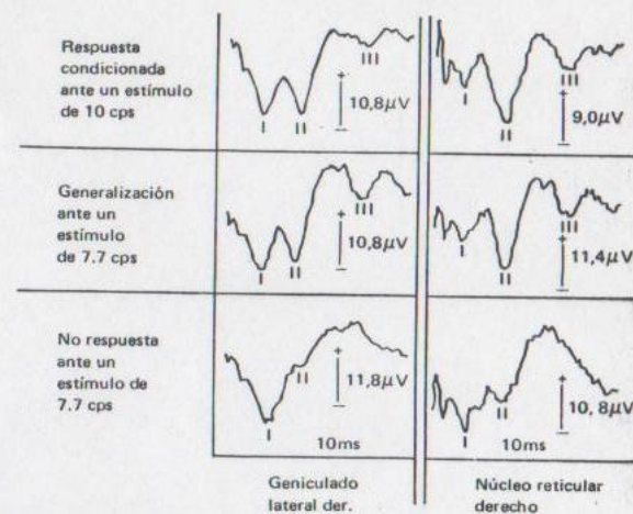
FIG. 3.10 Durante la respuesta condicionada ante un estímulo de 10 cps y la respuesta generalizada ante un estímulo de 7.7 cps, se registra la misma
