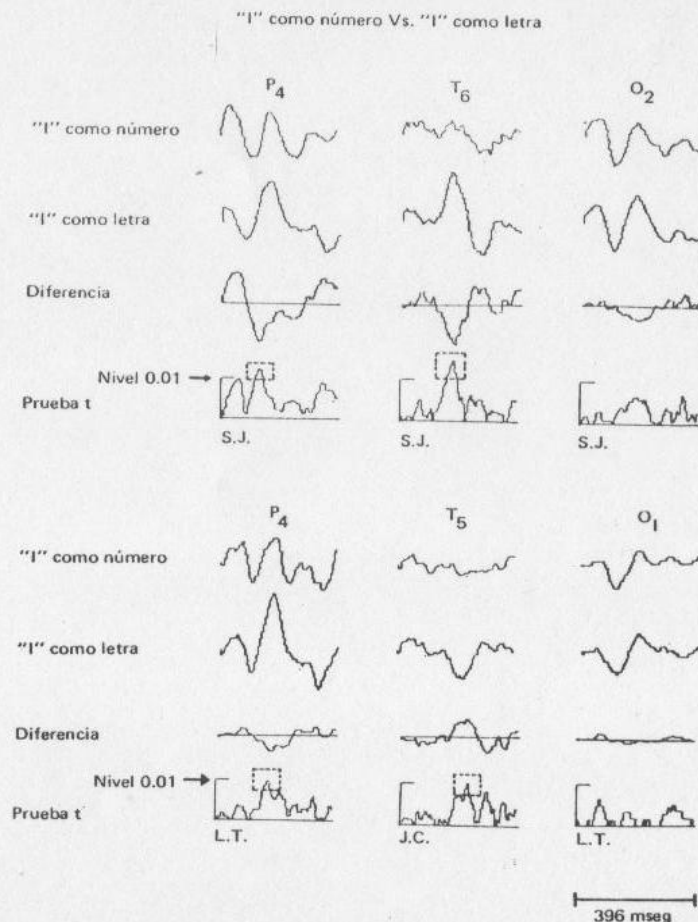
FIG. 3.16 Potenciales provocados, promediados con una computadora (100 muestras). El estímulo fue una línea vertical interpretada en 50% de los casos como un número 1 y en 50% de los casos como la letra I. Los potenciales provocados por la "letra" se restaron de los provocados por el "número" (Diferencia) y se obtuvo una prueba t. Solamente los registros de la zona parietal (P) y temporal (T 5 y T 6 ) difirieron. Los de la zona occipital no presentaron diferencias significativas. (Tomado de Grinberg-Zylberbaum y John, 1975.)
