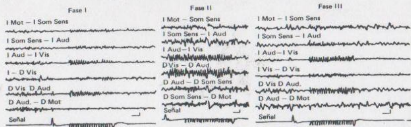
FIG. 3.3 Efectos del condicionamiento cortical sobre las respuestas electrofisiológicas ante un tono. La primera deflexión del canal de "señal" indica la aparición del tono. Después de dos segundos aparecen unos destellos a la frecuencia indicada en la señal. El tono y los destellos terminan juntos. Fase I: Desincronización generalizada de todas las áreas ante el tono. Fase II: Respuesta de frecuencia específica localizada en la corteza visual. Fase III: Desincronización específica localizada en la corteza visual. (Tomado de Morrell, 1961.)
