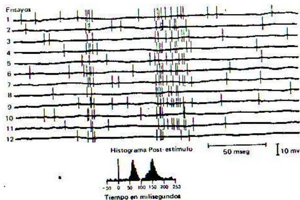
FIG. 4.4 Registros extracelulares de una neurona. Durante la aplicación de una barra negra sobre fondo luminoso (duración 50 msec.), la célula respondía con los patrones que se observan en la porción superior de la figura (cada uno de los 12 patrones representa sendas presentaciones del estímulo). Mediante una computadora se obtuvo el histograma de frecuencias que se muestra en la parte inferior. Los dos picos del histograma reflejan los dos incrementos en la frecuencia de disparo de la unidad que se observan en los registros superiores. (Tomado de Morrell, 1967.)
