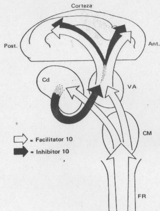
FIG. 2.7 "Círculo del caudado" mostrando las influencias facilitadoras e inhibitorias entre sus componentes. Cd.: núcleo caudado; V.A.: núcleo ventral anterior; C.M.: núcleo centro mediano; R.F. formación reticular. (Tomado de Buchwald y colaboradores, 1961.)
